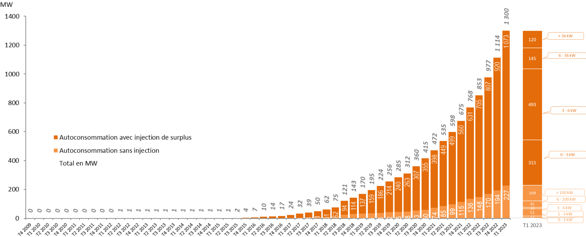
Cumul des raccordements par trimestre en MW – France continentale
